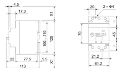
CLW1-40 ... CLW1-80
