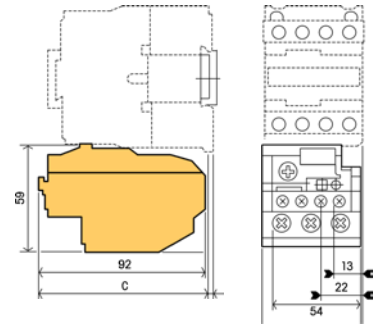
CLY1-B (CLZ2-F)
