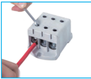
Conexión de cableado Wire connection
