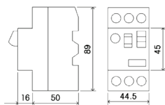
CLW1-01 ... CLW1-32
