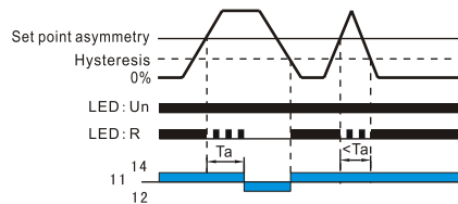
Protección asimétrica
